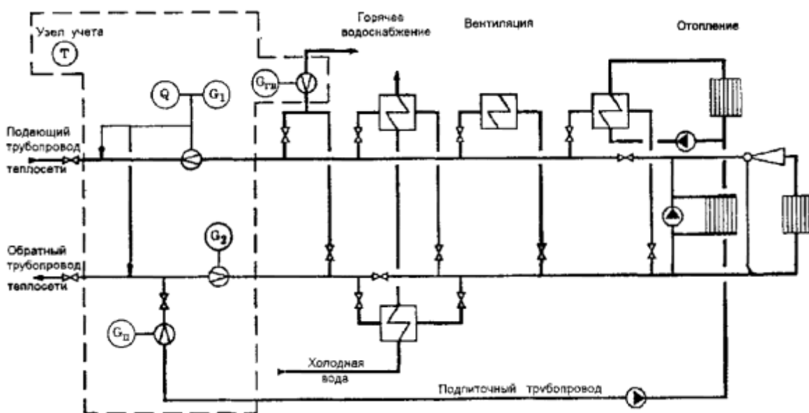
Рис. 5. Принципиальная схема размещения точек измерения количества тепловой энергии и массы (объема) теплоносителя в открытых системах теплоснабжения с суммарной тепловой нагрузкой, не превышающей 0,5 Гкал/ч
